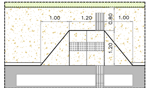
DETALHE – RAMPA ESCALA – 1:75
